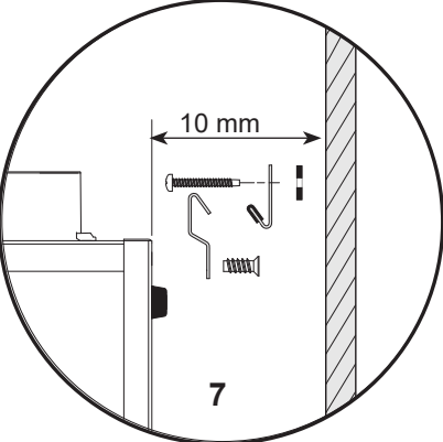
Montage muurophangset
